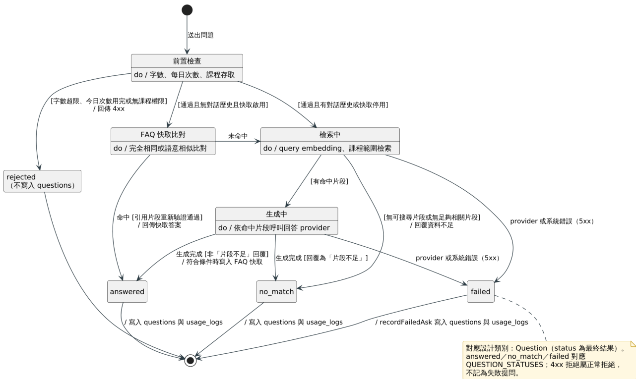
QA提問狀態機圖
