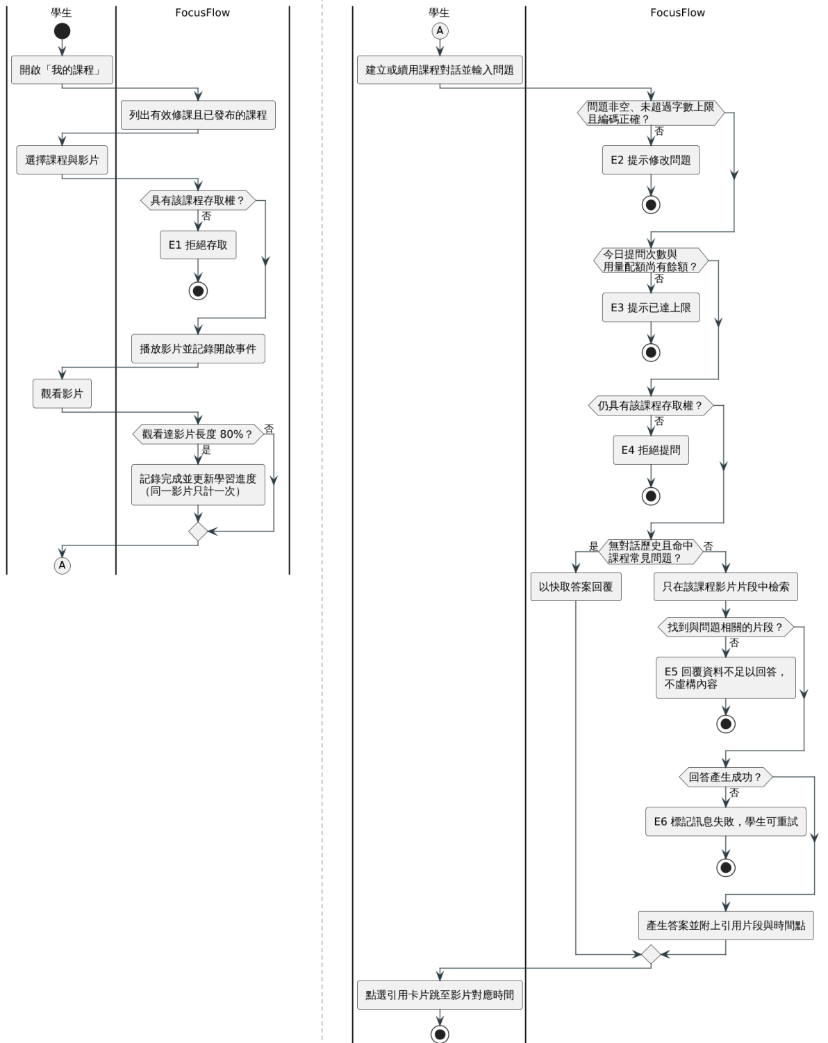
學生網頁觀看與提問活動圖
