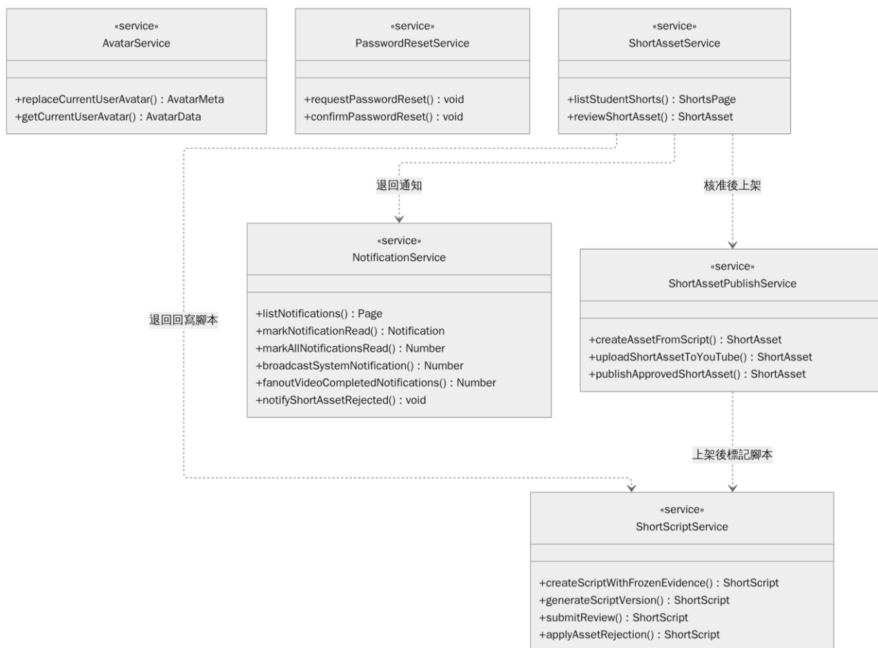
圖 6-2-3a 個人資料通知與短影音服務設計類別圖
