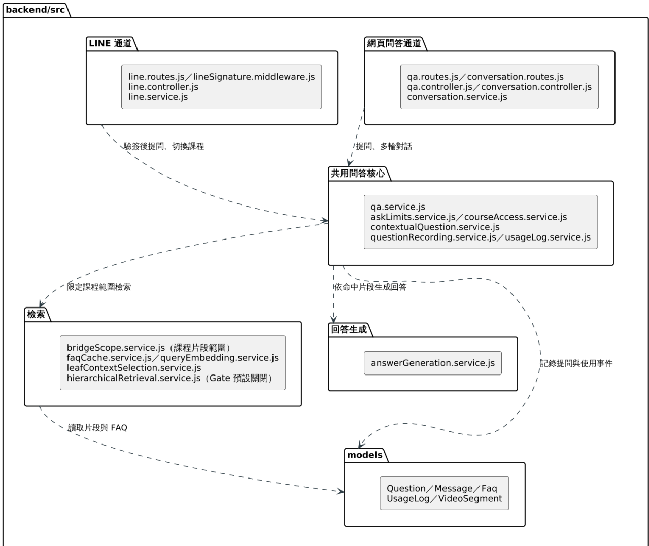
LINE與QA套件圖
