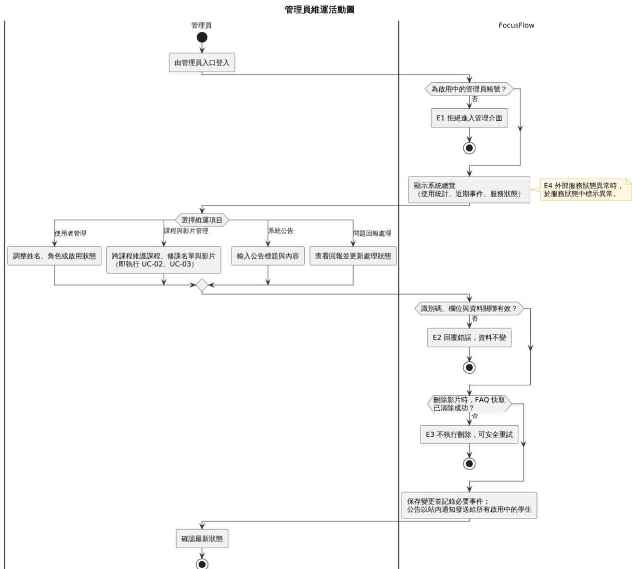
圖 5-3-9 管理員維護活動圖
