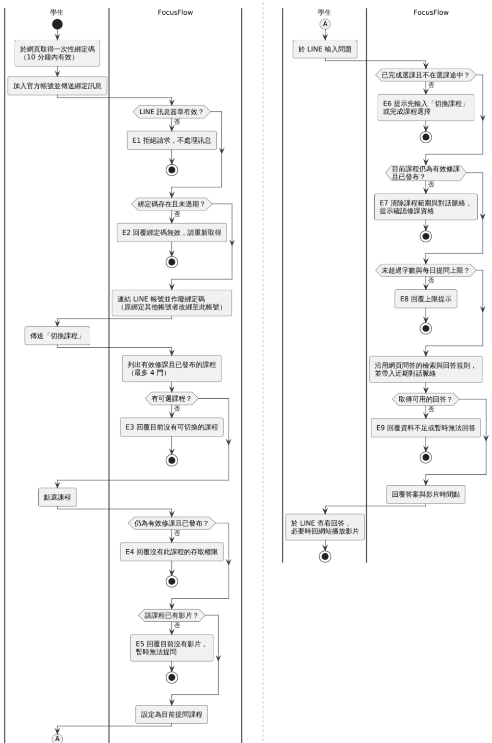
LINE綁定與課程問答活動圖
