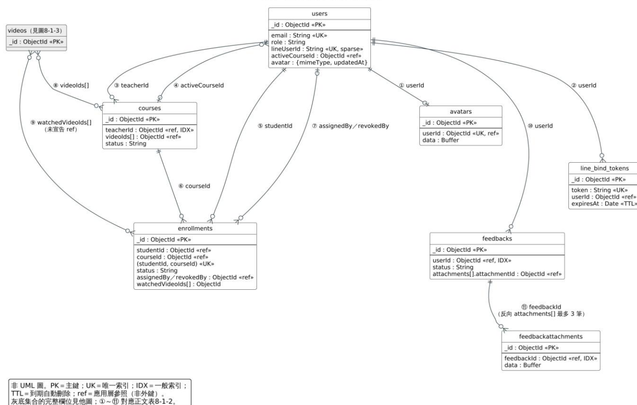
帳號、課程與問題回報集合關聯圖
