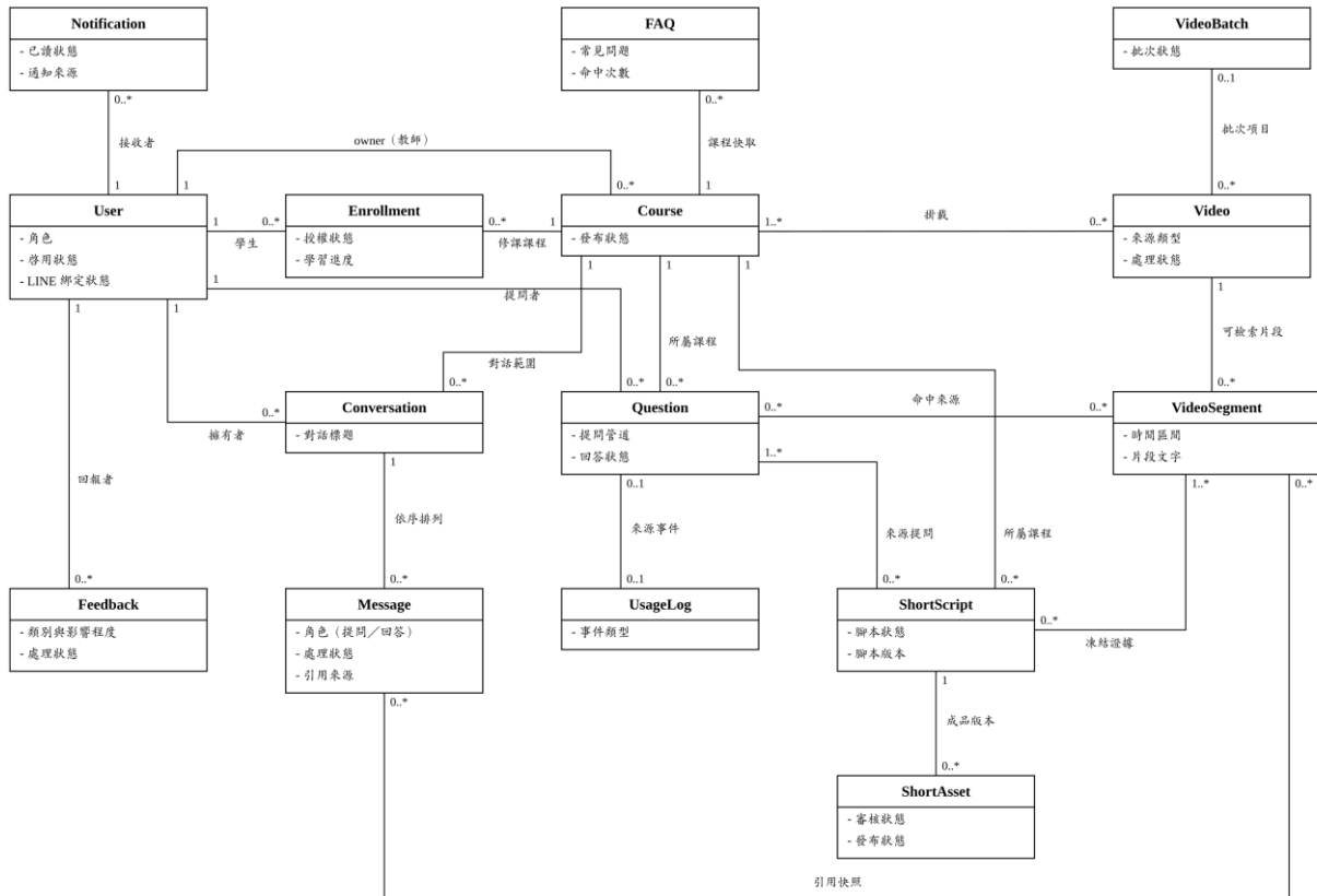
系統分析類別圖
