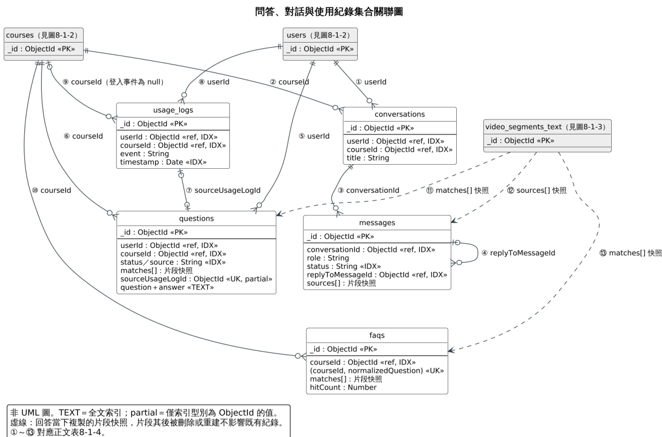
圖 8-1-4 問答、對話與使用紀錄集合關聯圖
