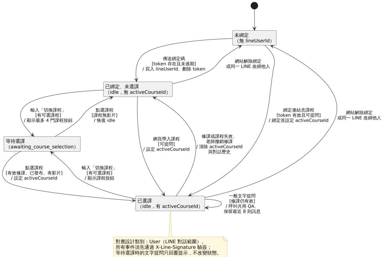
LINE對話範圍狀態機圖
