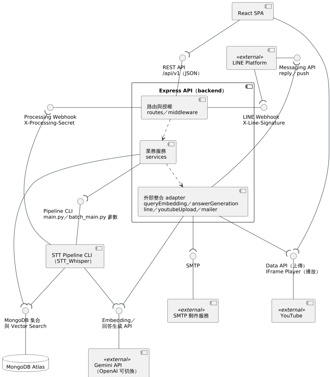
系統元件圖
