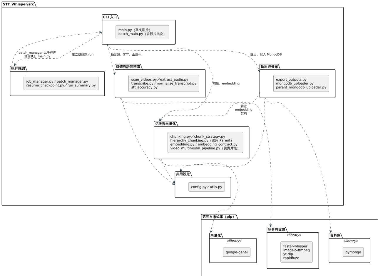
AI-Pipeline套件圖
