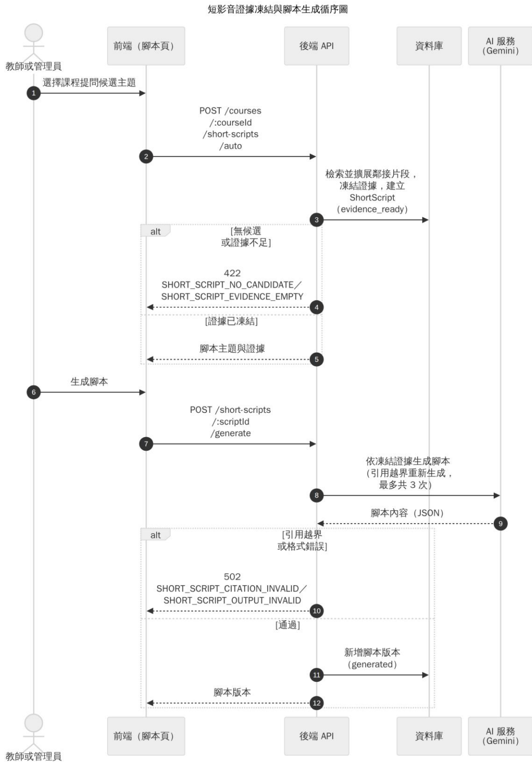
圖 6-1-8a 短影音證據凍結與腳本生成循序圖
