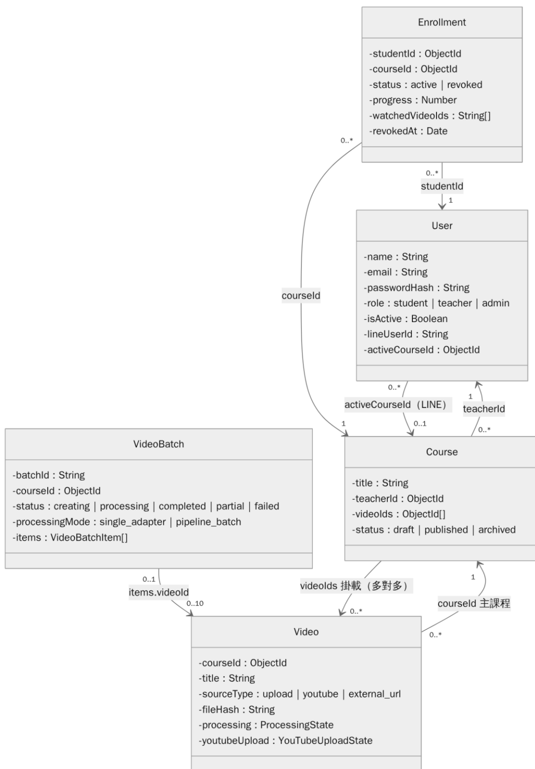
圖 6-2-1b 帳號課程與影片資料設計類別圖
