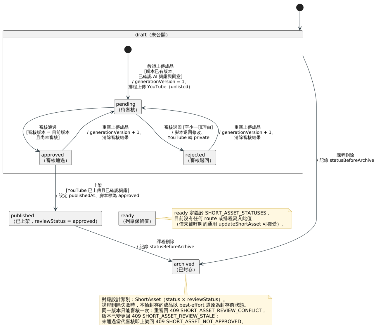
短影音成品狀態機圖
