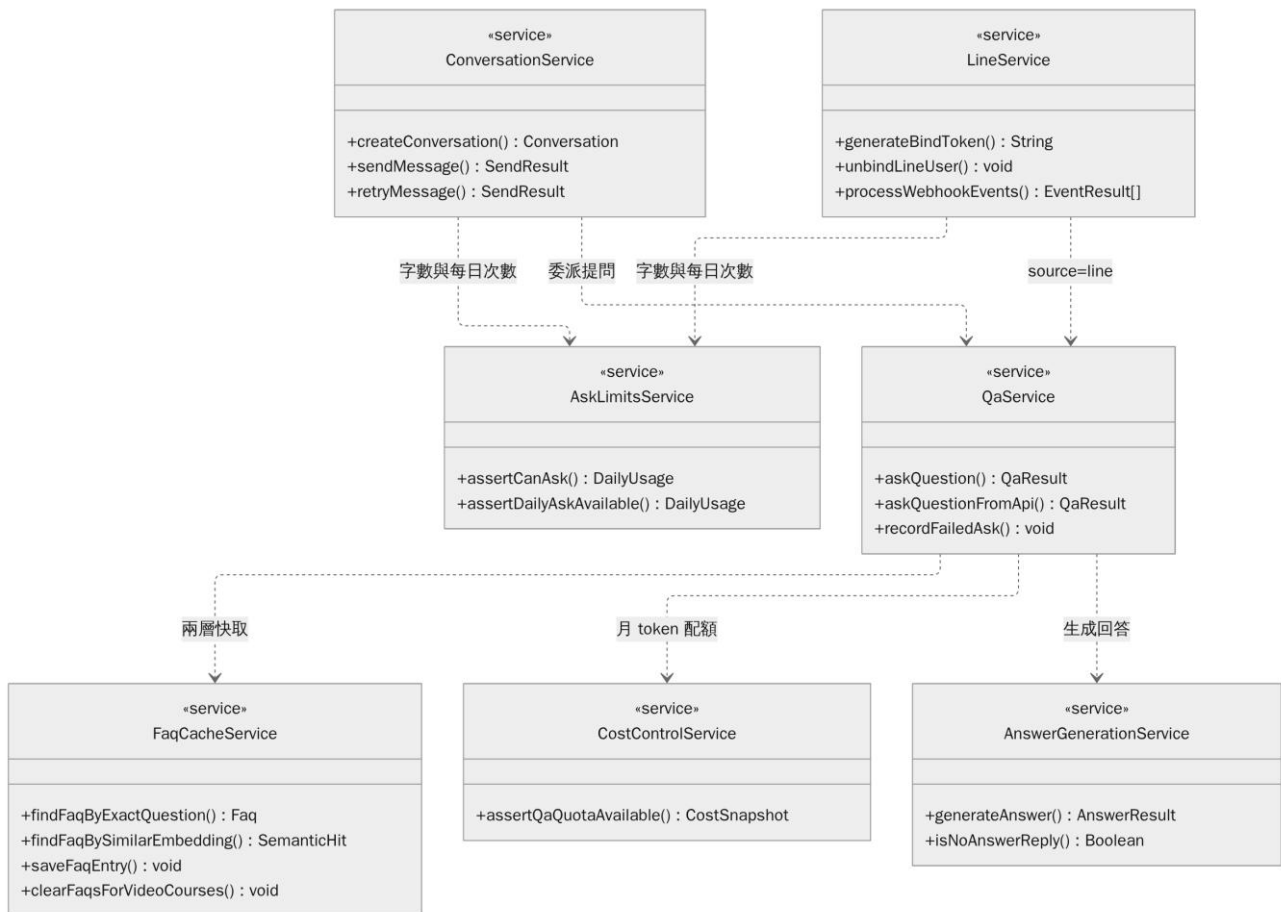
問答與對話服務設計類別圖
