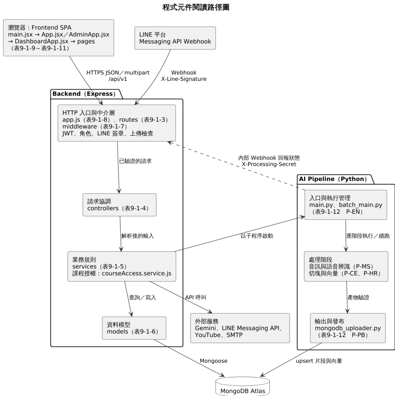
圖 9-1-1 程式元件閱讀路徑圖
