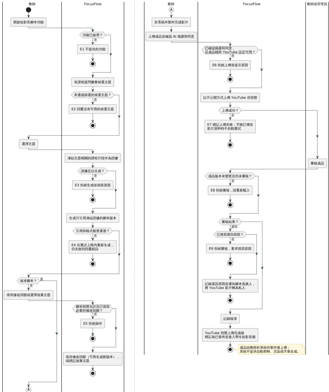
短影音腳本與成品審核活動圖
