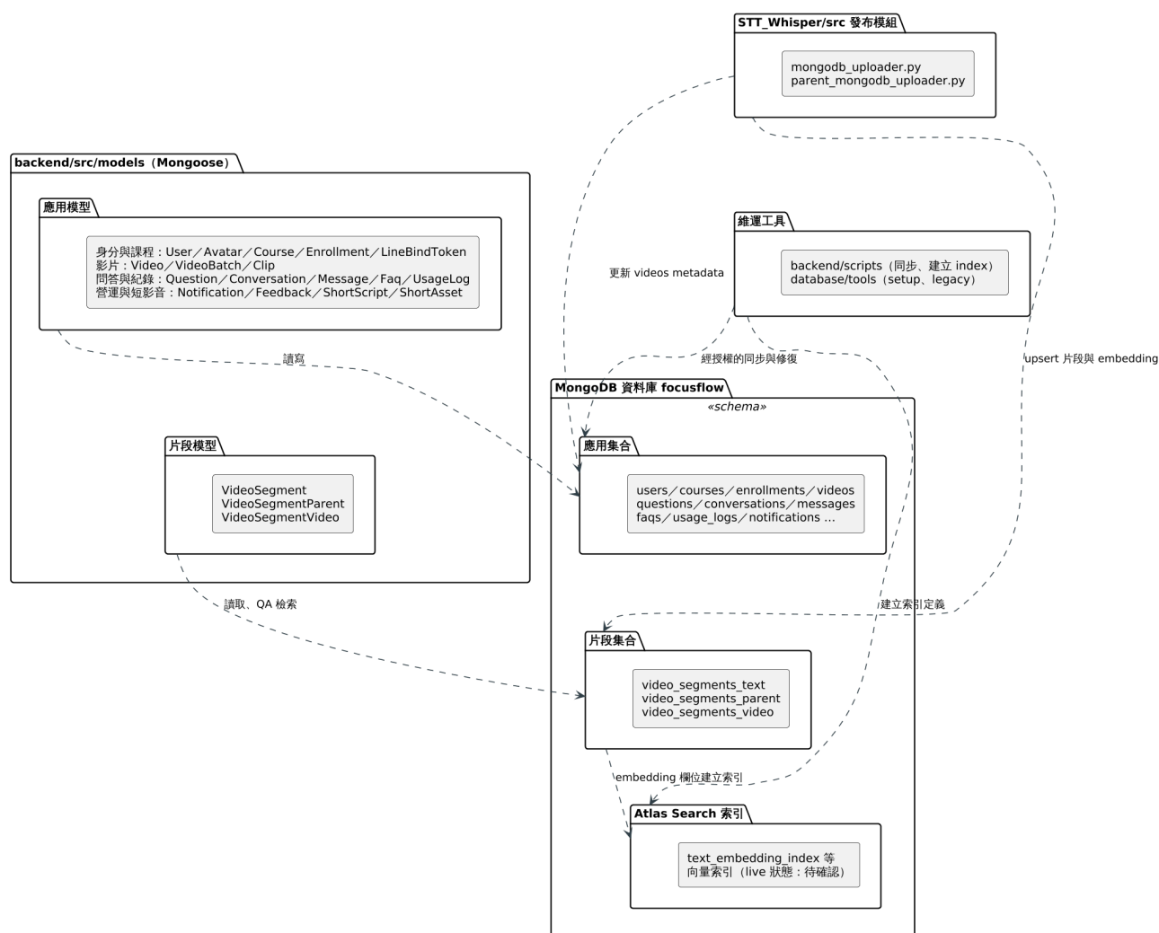
資料儲存套件圖
